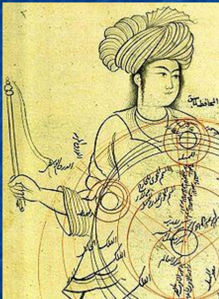
Манускрипт Кутб ад-Дина аш-Ширази, иллюстрирующий его теорию планетных движений.
